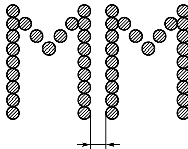
Рисунок 5 — Интервал между знаками
