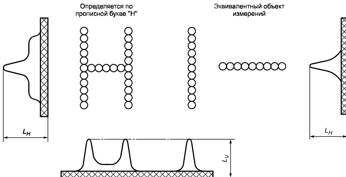
Рисунок 15 — Однородность яркости внутри знака
