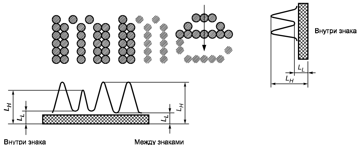
Рисунок 16 — Яркостный контраст внутри знака и между знаками и траектории перемещения фотометра
