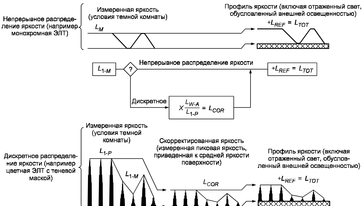
Рисунок 10 — Профили яркости для измеренной, скорректированной и полной яркости
