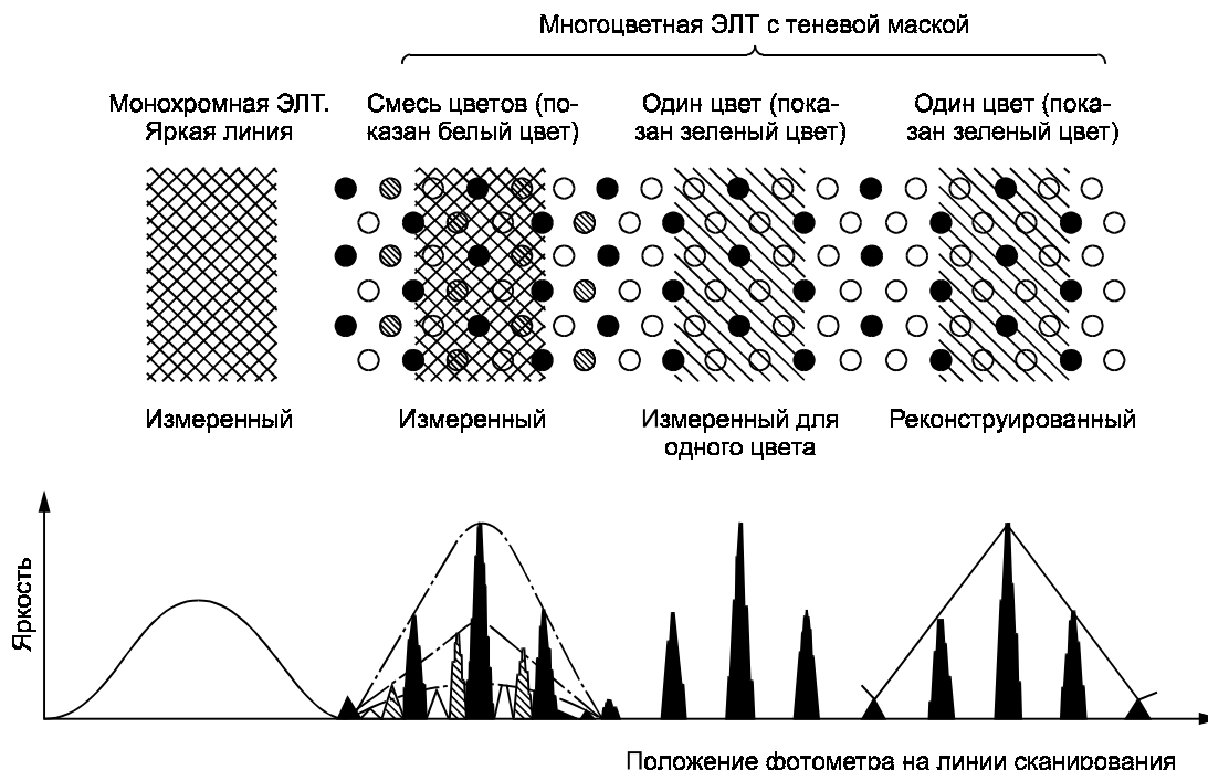
Рисунок 8 — Измеренные и реконструированные профили яркости
