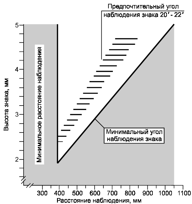
Рисунок 1 — Соотношение между проектным расстоянием наблюдения и высотой знака
