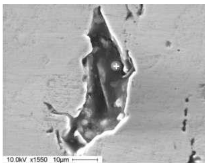
Рисунок 9. Характерные неметаллические включения в заготовках стали 09Г2С: а – \text{Al}_2\text{O}_3 \cdot \text{SiO}_2 ; б – \text{FeO} \cdot \text{SiO}_2
