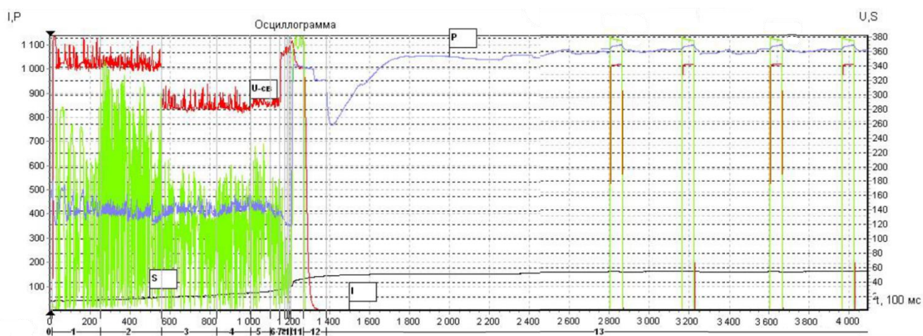
Рисунок 6. Осциллограмма сварки образца 4
