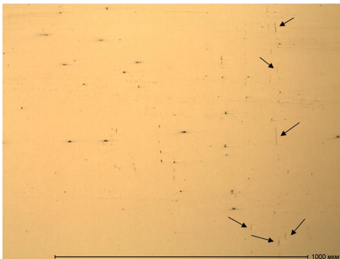
Рисунок 7. Силикаты пластичные на заготовках от плавков стали 09Г2С, произведенных по стандартной технологии
