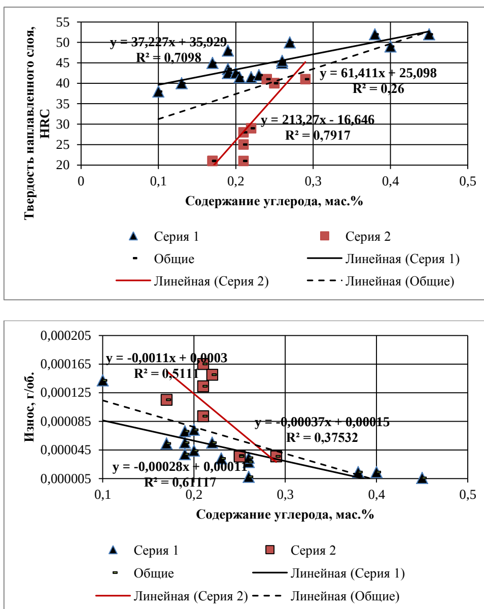
Рисунок 1. Влияние содержания углерода на твердость и износ
