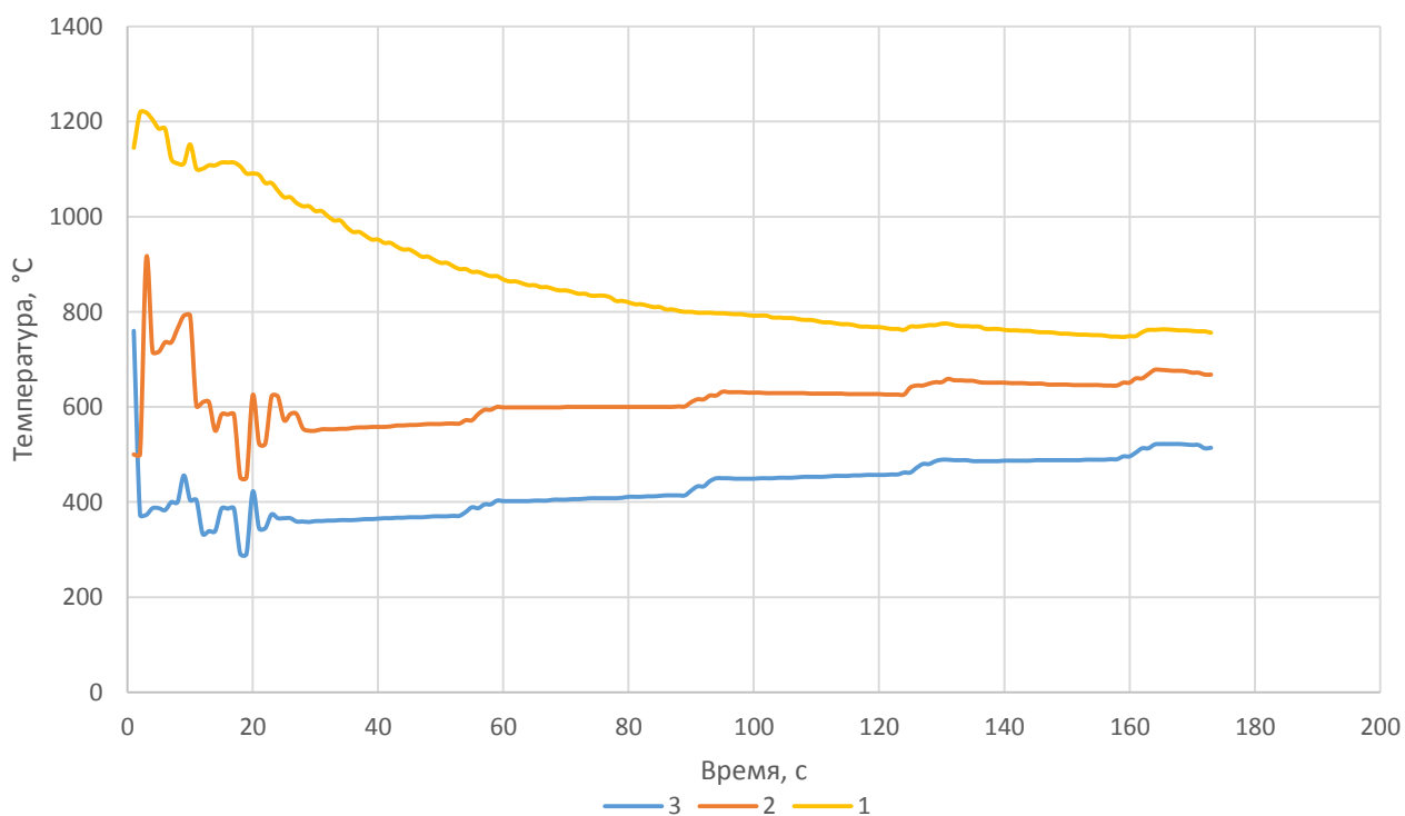
Рисунок 15. График охлаждения после сварки образца 10
