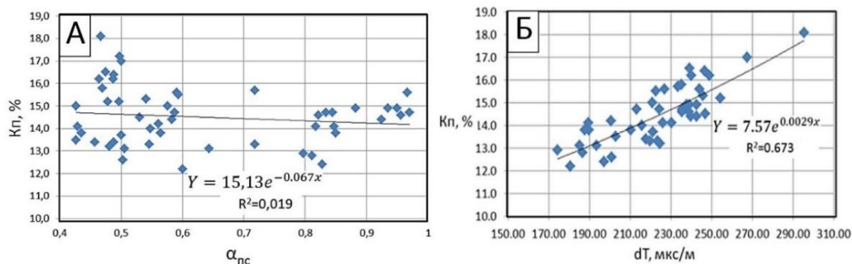
Рисунок 3. Теснота корреляционной связи коэффициента пористости ( K_{п} ) пласта Ю_1^{1-2} и относительной амплитуды ПС ( \alpha_{пс} ) (А), K_{п} и интервального времени ( dT ) (Б). Поля корреляции по 29 скважинам
